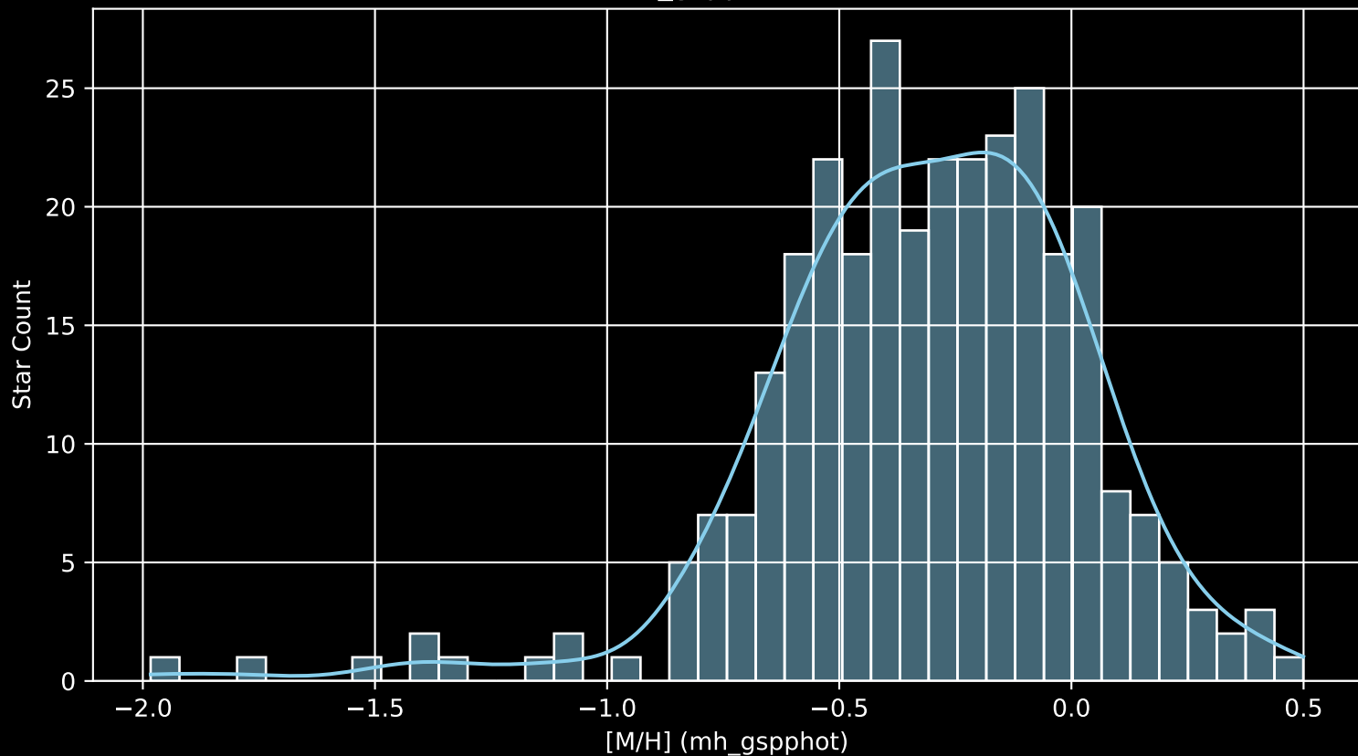
GALAH DR4 Field: [6923] [M/H] (mh_gspphot) (n= 305)
