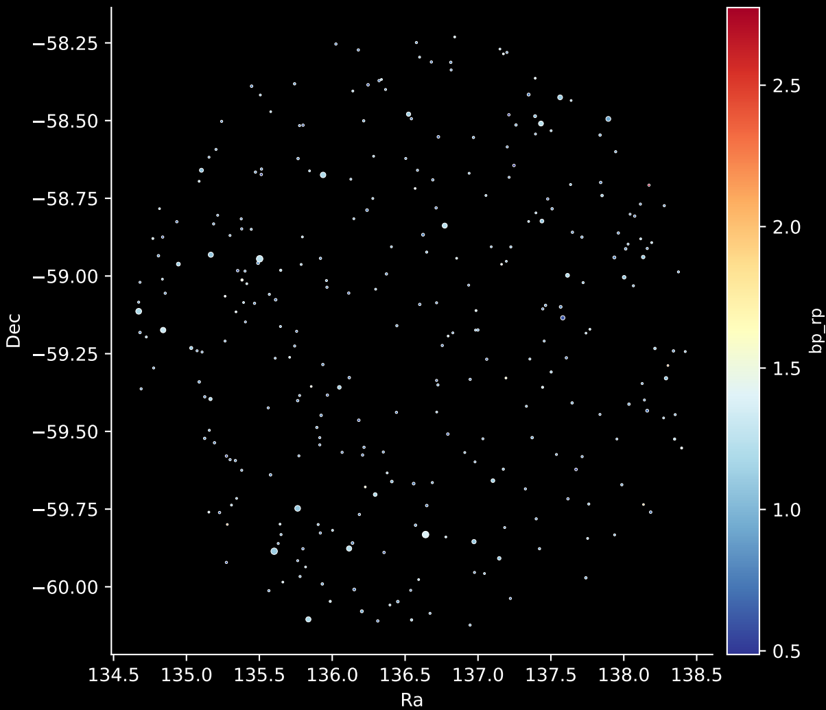
GALAH DR4 Field: [6923] Stars: 305
