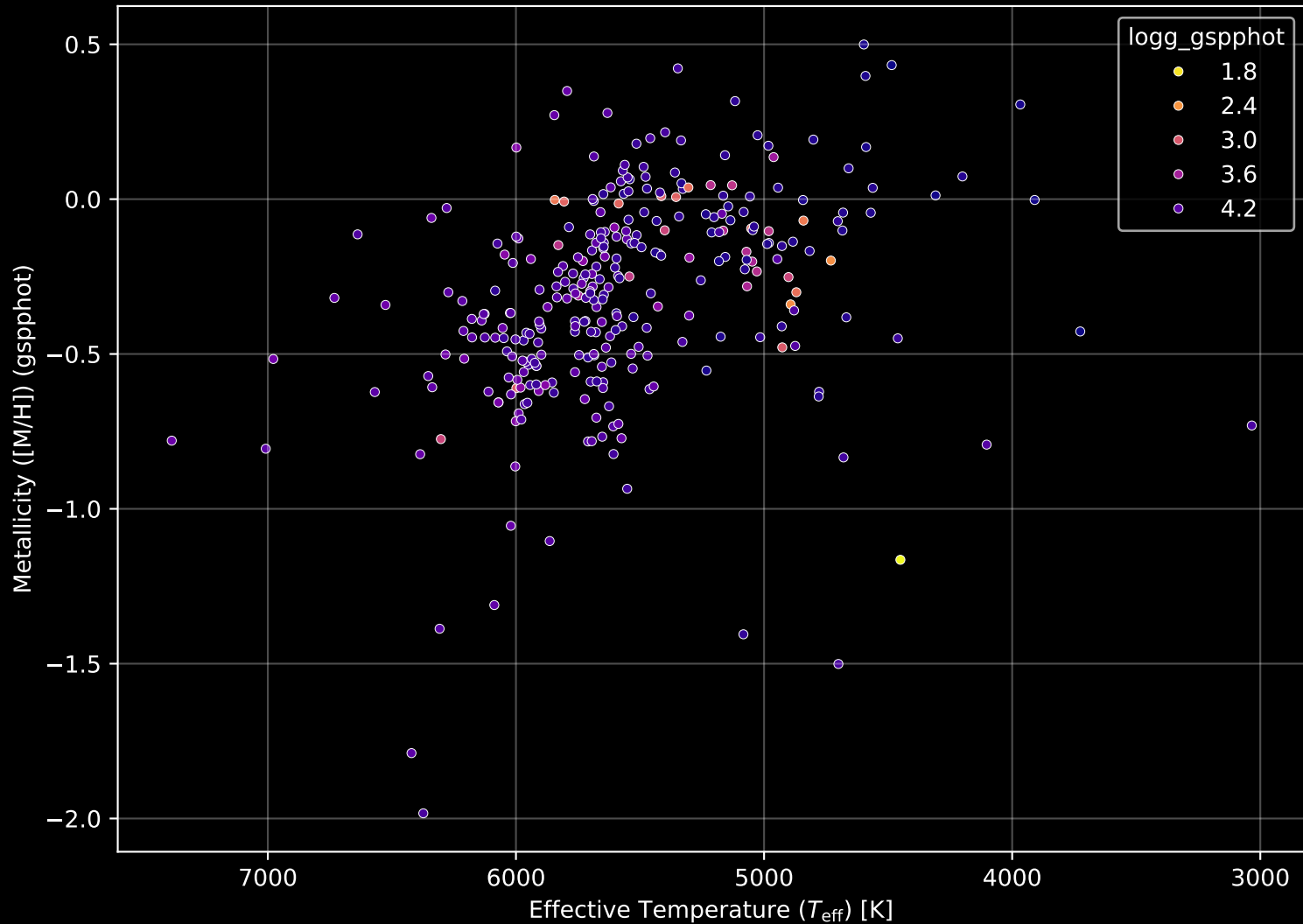
GALAH DR4 Field: [6923] Stellar Population Parameters (n= 305)
