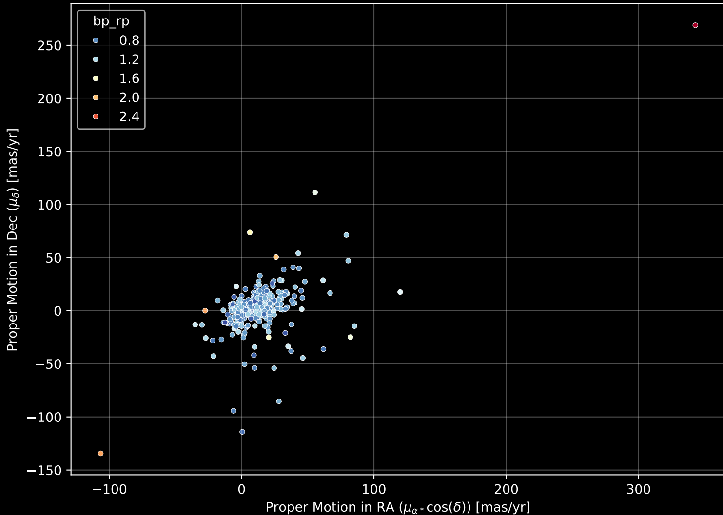
GALAH DR4 Field: [6923] Proper Motion Diagram (n= 305)
