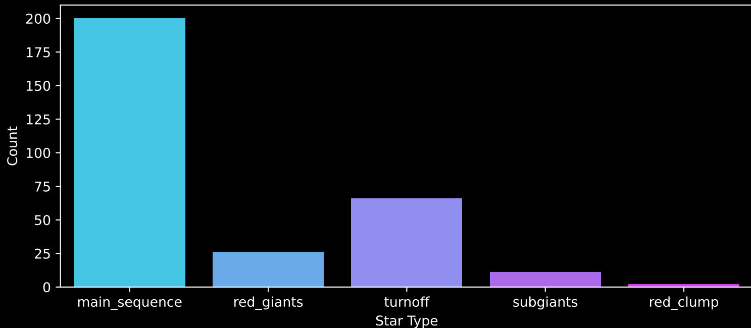
GALAH DR4 Field: [6923] Count plot of Star Type
