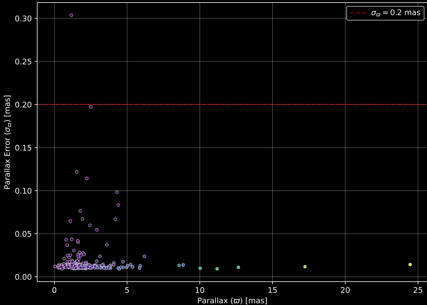
GALAH DR4 Field: [6923] Parallax Quality (n= 305)
